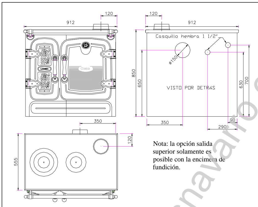
Figura nº1 – Dimensiones en mm Cocina Clásica 7TE.
