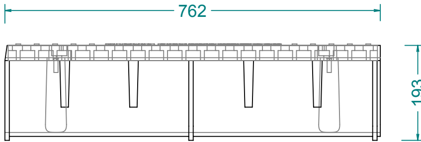
vista alzado 1:10
