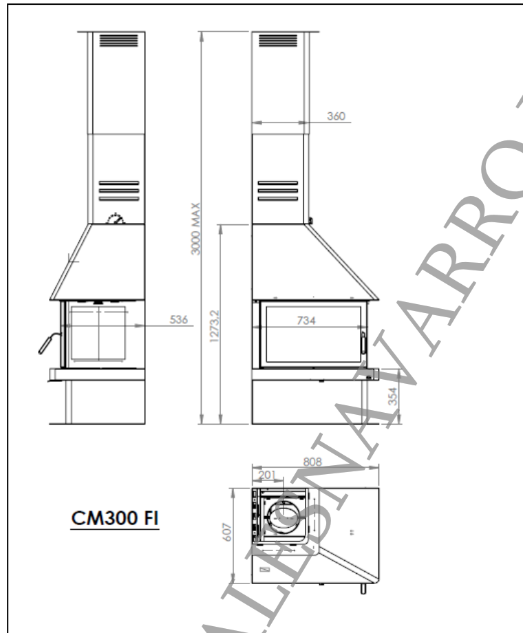
Figura nº3 – Dimensiones CM300FI en mm
