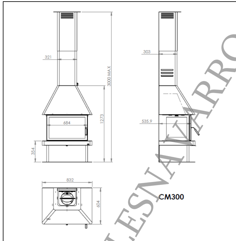
Figura nº1 – Dimensiones CM300 en mm
